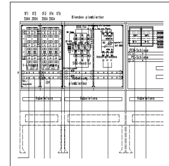
Aufbauplanansicht Teilbereich
